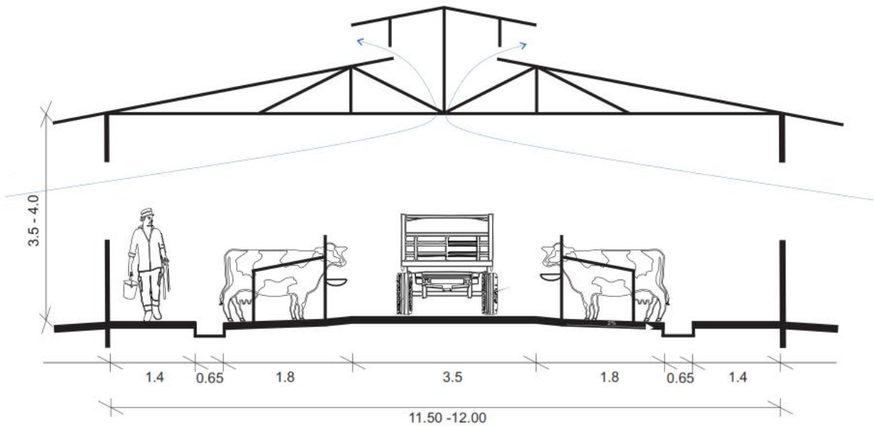
სურათი 2: სადგომის გვერდითი ქრილი.
